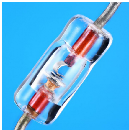
Fotografia spínacej diódy v sklenenom púzdre
