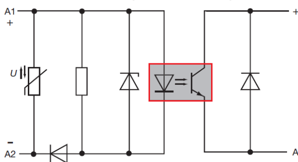
Zapojenie optronu v elektrickom obvode
