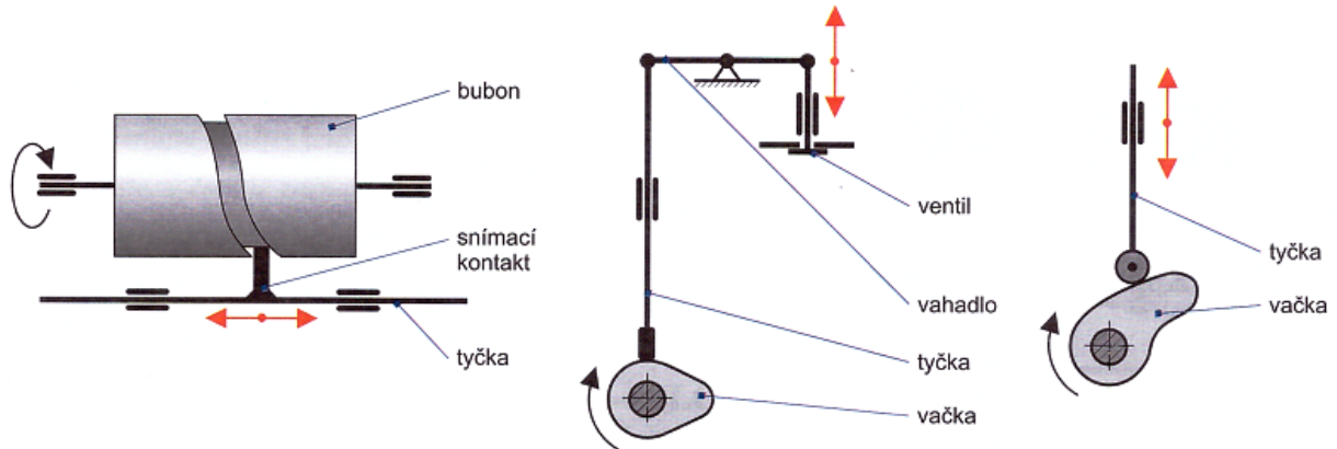
Vačkové mechanizmy
