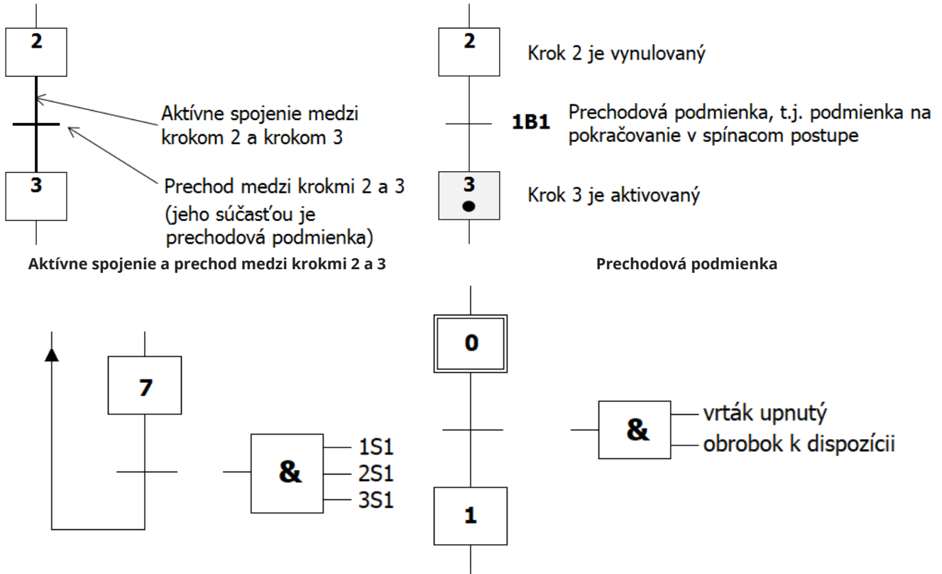
Príklady prechodovej podmienky inak Grafcet
