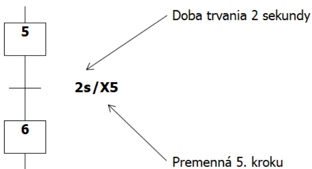
Príklad časovo závislého prechodu, časovo závislej prechodovej podmienky
