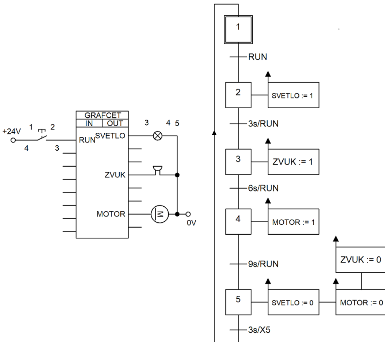
Príklad podmienky realizujúcej prechod na ďalší krok programu až po stlačení tlačidla trvajúcom dlhšie ako 3 sekundy, 6 sekúnd, 9 sekúnd...
