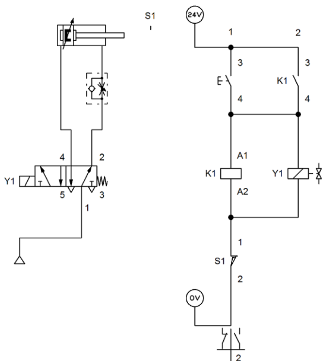
Elektro-pneumatická schéma
