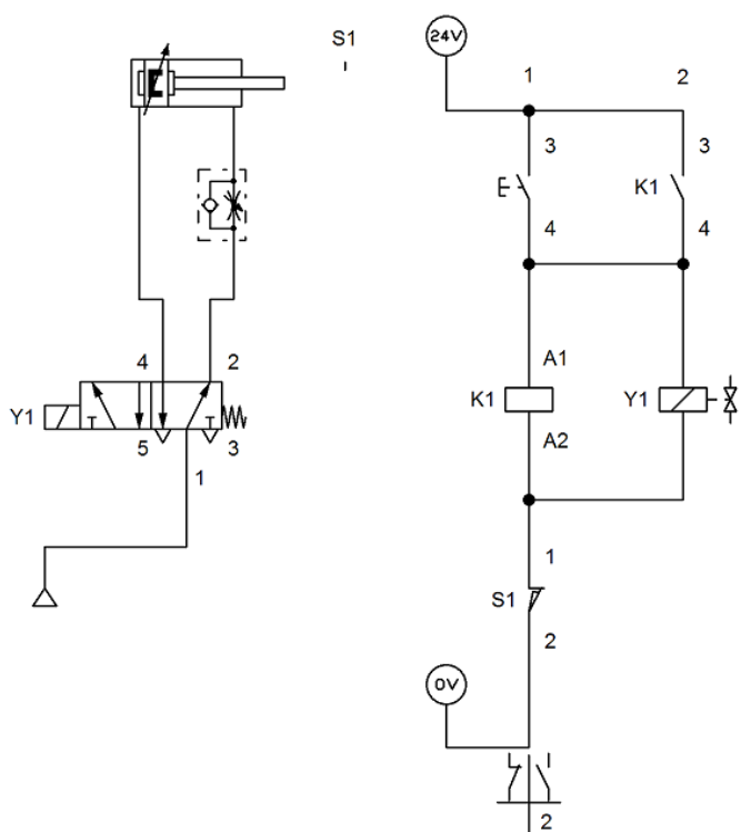
Elektro-pneumatická schéma
