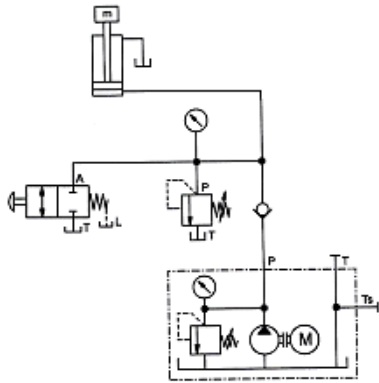
Hydraulická schéma
