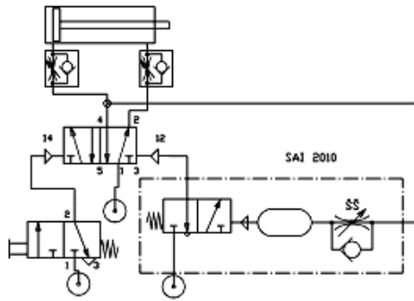
Pneumatická schéma
