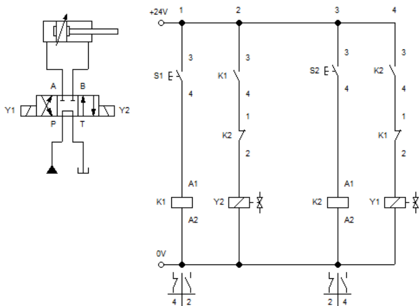
Elektro-hydraulická schéma
