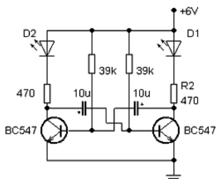
Elektronická schéma
