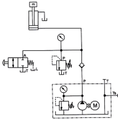
Hydraulická schéma
