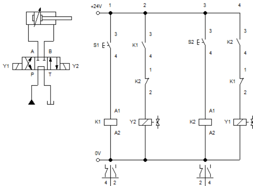
Elektro-hydraulická schéma
