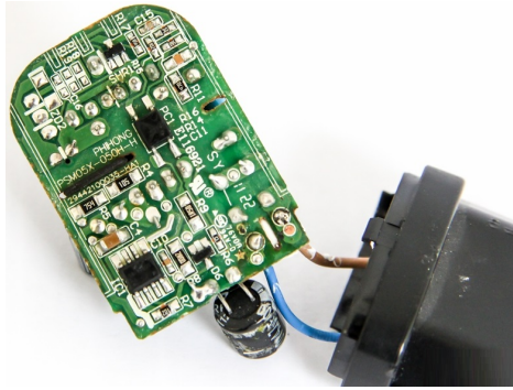
SMD technológia použitá v nabíjačke
