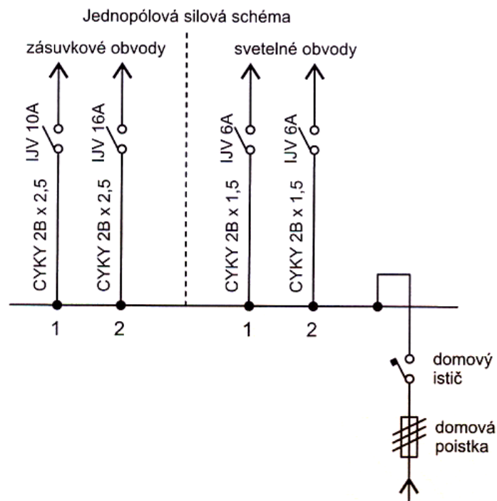
Schéma zapojenia hlavného rozvádzača
