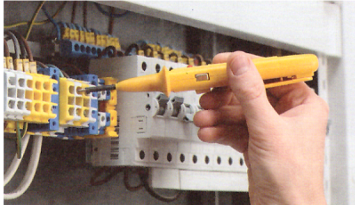
Hlavný rozvádzač
