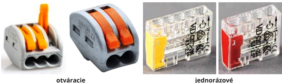
Wago svorky
