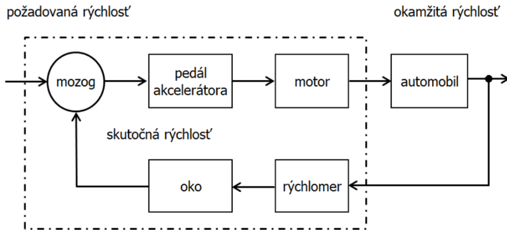
Príklad regulácie rýchlosti idúceho automobilu
