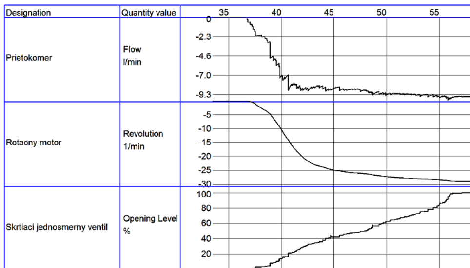
Meranie prietoku v pneumatike
