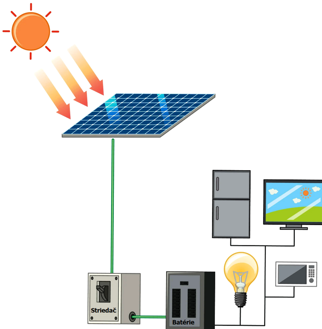
Ostrovný fotovoltaický systém
